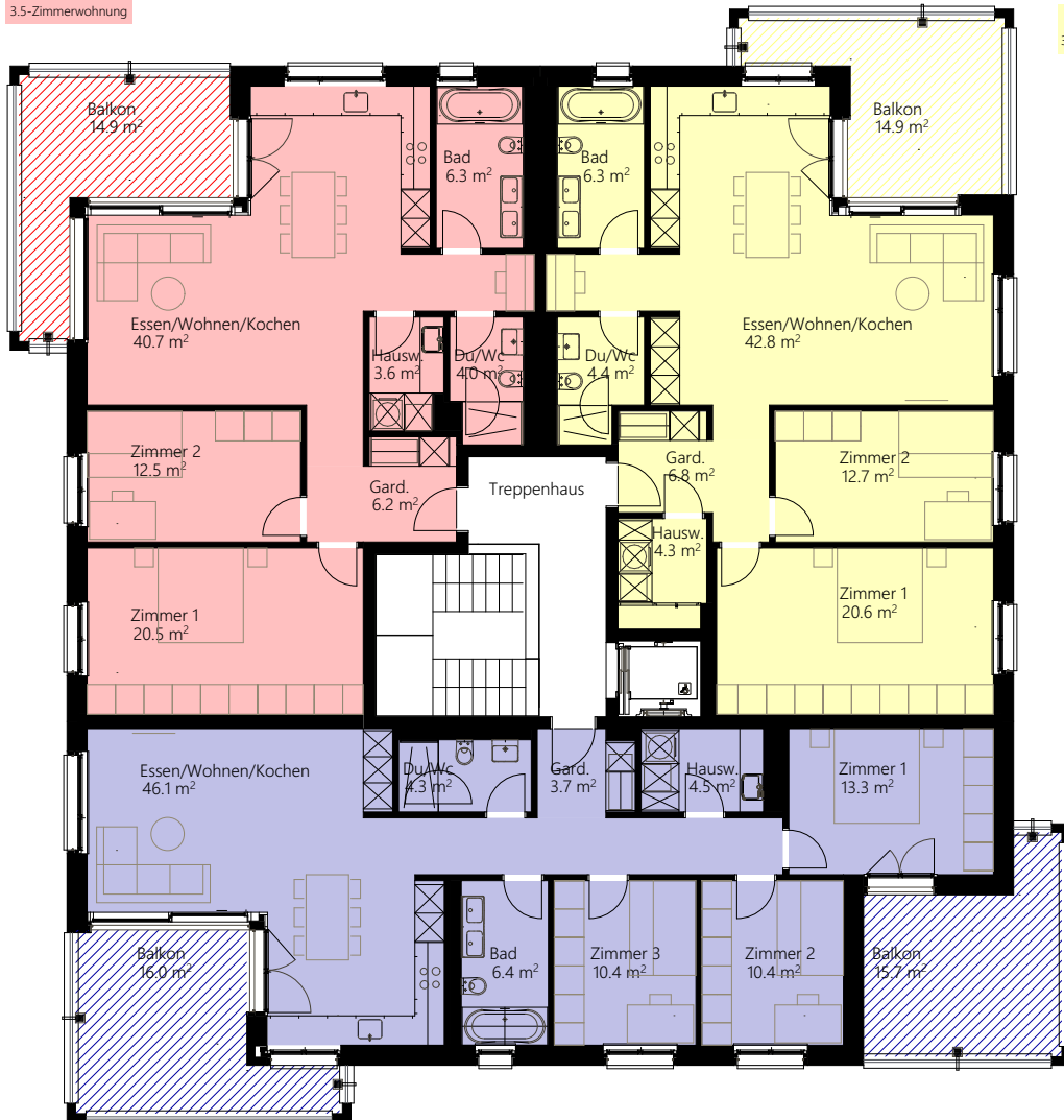
S-2-W08 98.3 m 2 4.5-Zimmerwohnung
